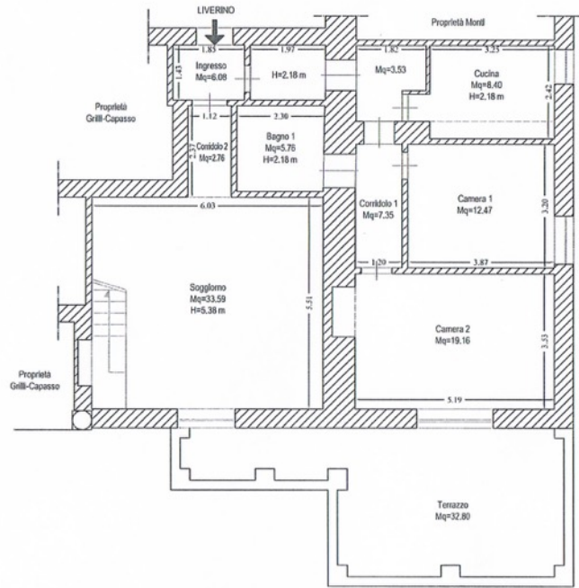
Pianta Piano Primo Rapp. 1:100
